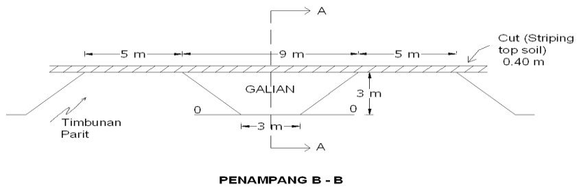
Penampang B-B
