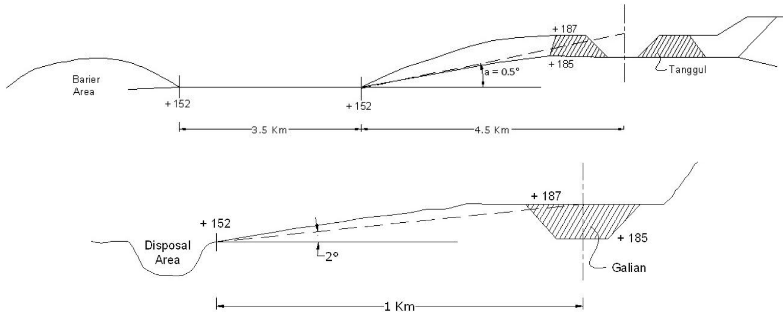
Gambar II.C.2 Penampang potongan lokasi pembuatan saluran dan tanggul
